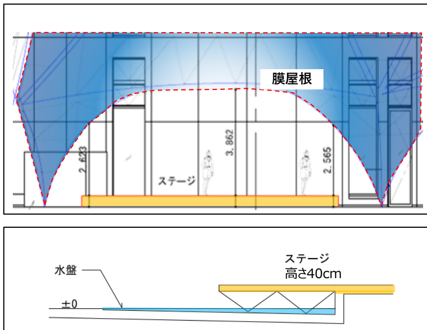
(ステージ立面図)
